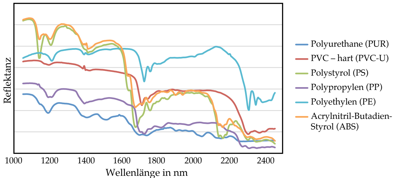
Mittlere Punktspektren verschiedener Kunststoffe
