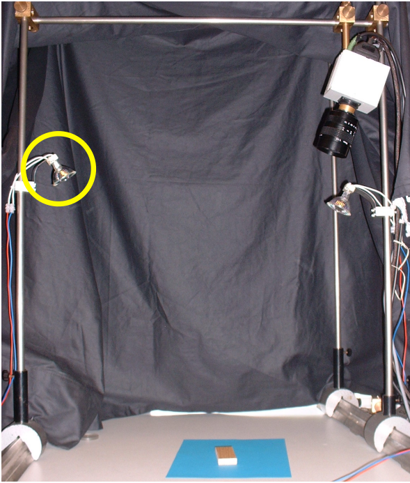
Messaufbau
