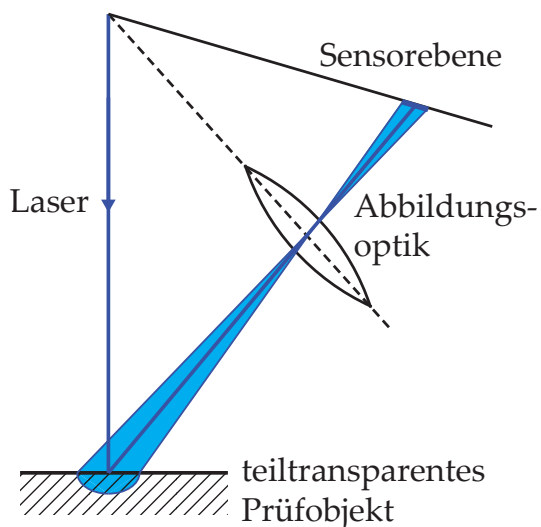
Aufweitung des Lichtpunktes durch teiltransparentes Objekt
