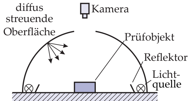
Diffuse Beleuchtung mit Hilfe eines halbkugelförmigen Schirms
