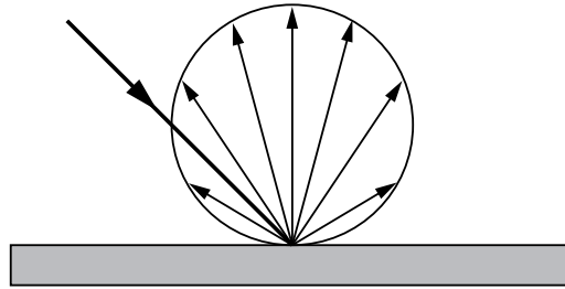
Lambert'sche Streuung
