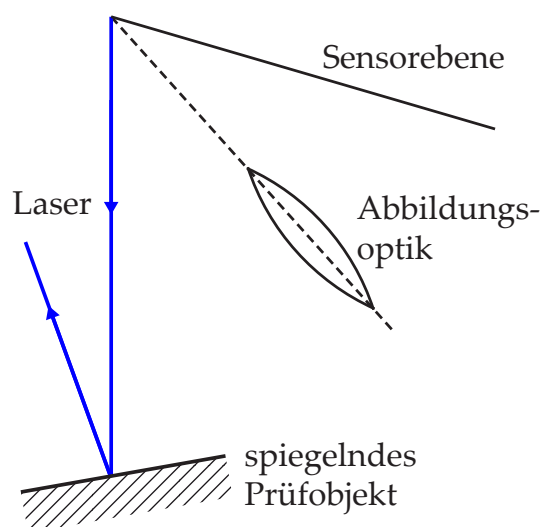
Bei perfekt spiegelnden Objekten gelangt kein Licht auf den Detektor
