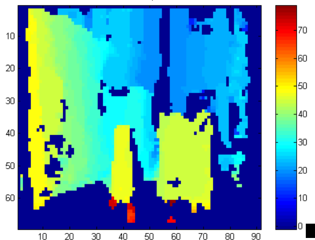
Gefilterte Disparität
