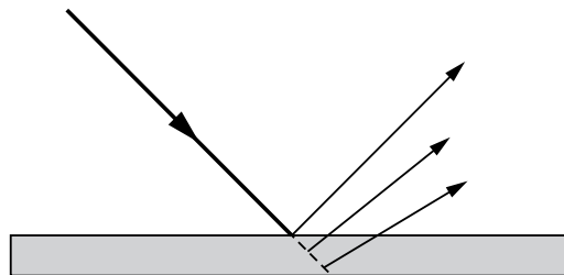
Volumenstreuung
