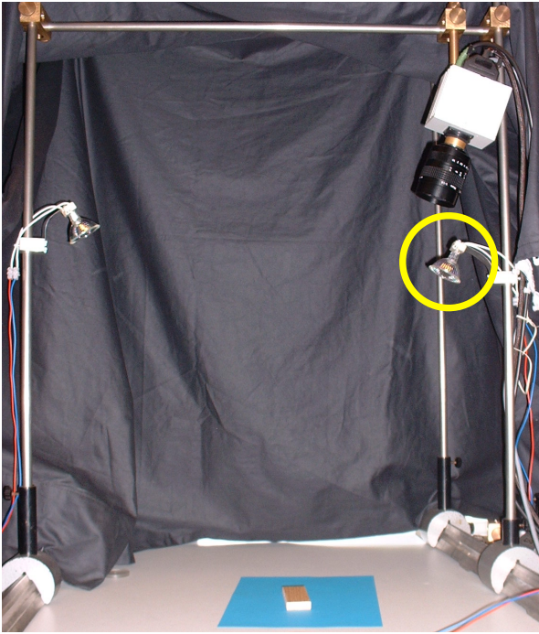
Messaufbau
